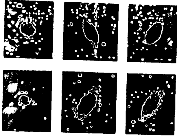
أنواع من المجرات
